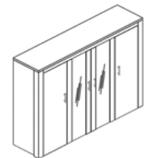
6MA.110810 176x43x143H
